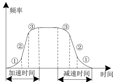
图 6-4 S 曲线加减速
