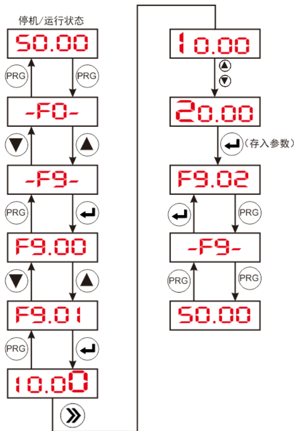
图 4-2 三级菜单操作流程图
