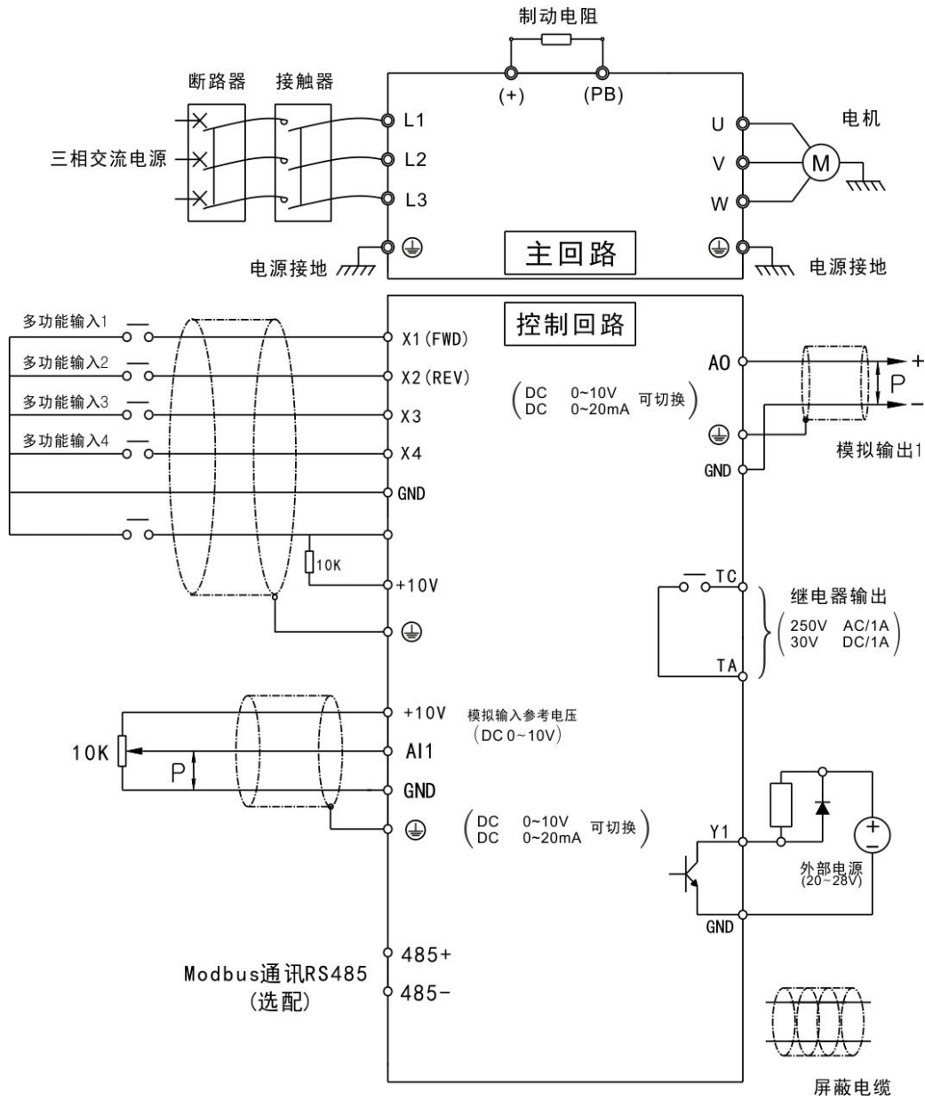
图 3-2 Commander XL 系列基本配线图
