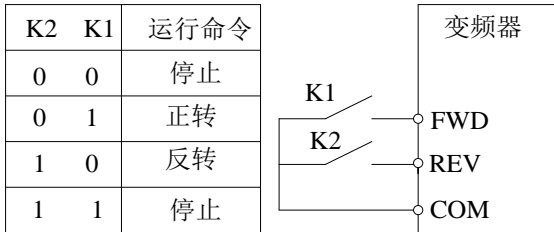
图 6-14 两线式 1
