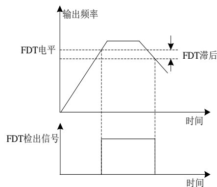
图 6-22 FDT 电平示意图
