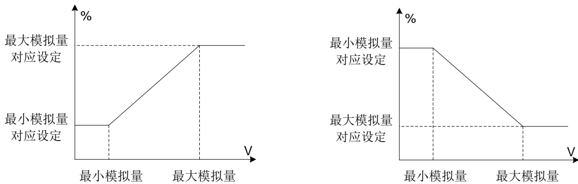
图 6-19 模拟输入线性曲线
