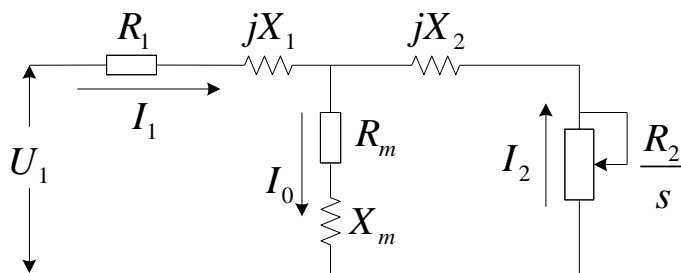
图 6-13 异步电机稳态等效电路图
