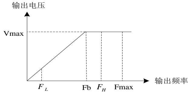
图 6-1 输出频率与输出电压关系图
