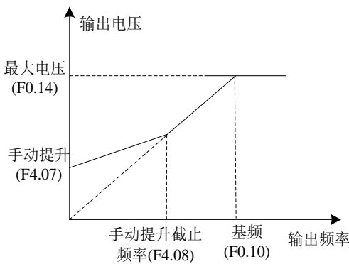
图 6-11 转矩提升
