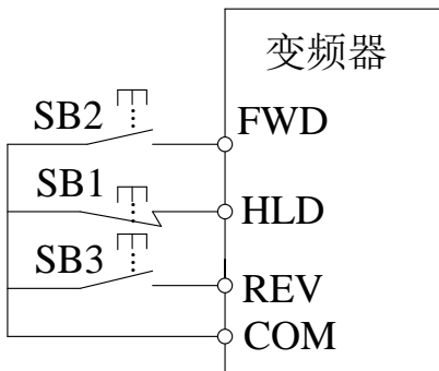
图 6-16 三线式 1
