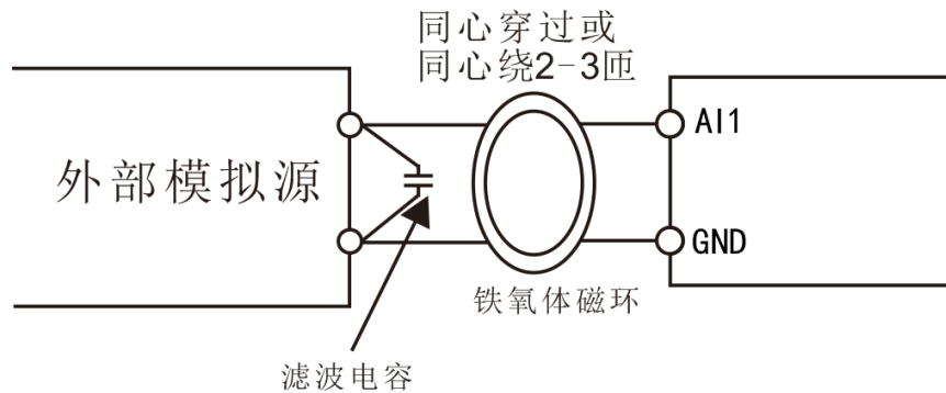
图 3-5 模拟输入端增加滤波器接线示意图
