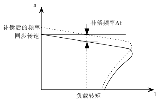
图 6-12 自动转差补偿
