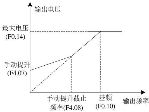
图 6-11 转矩提升
