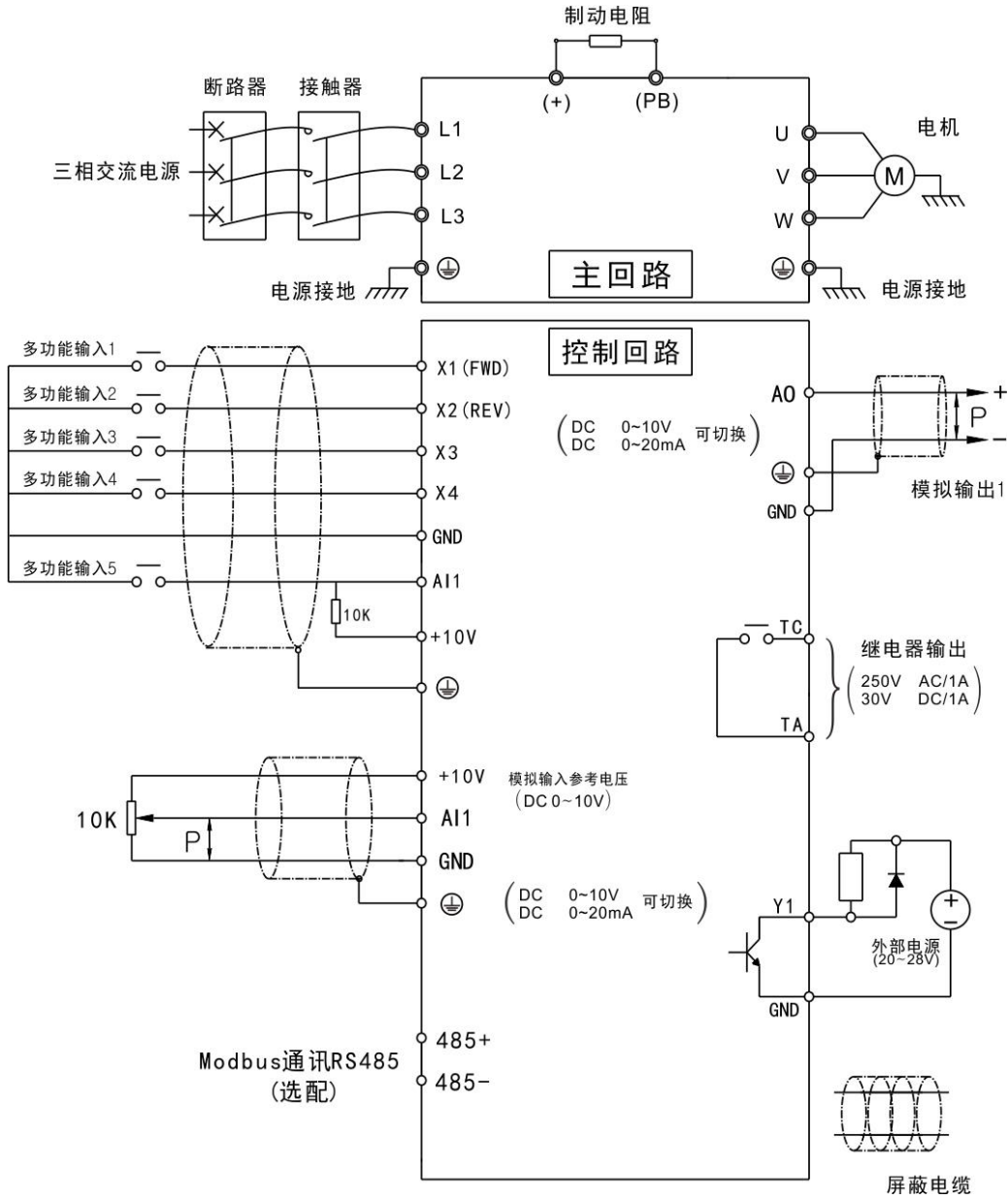
图 3-2 COMMANDER X 系列基本配线图
