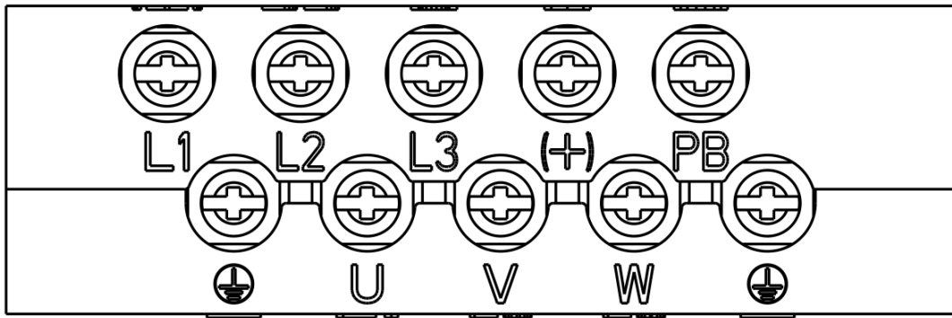
图 3-3 COMMANDER X 系列主回路端子配线图
