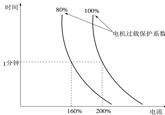
图 6-28 电机过载保护系数设定
