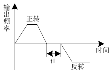
图 6-6 正反转切换
