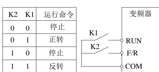
图 6-15 两线式 2
