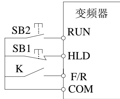
图 6-17 三线式 2
