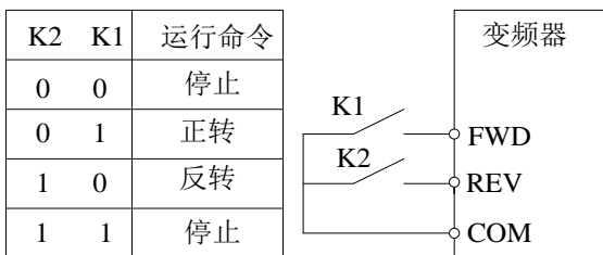
图 6-14 两线式 1
