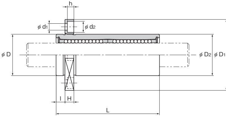
LMIK-L型
