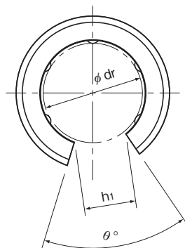
LM-OP型
