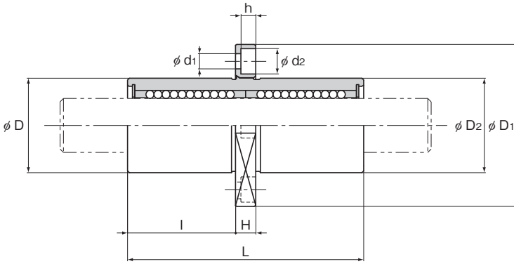
LMCK-L型
