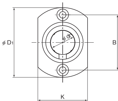
LMIH 6L~13L型
