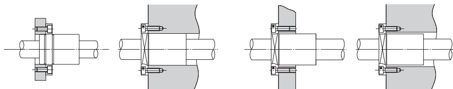
配合方式安装轴承套
