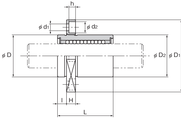
LMIK型
