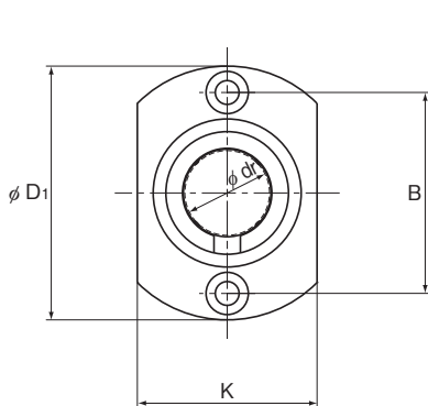
LMIH 6~13型
