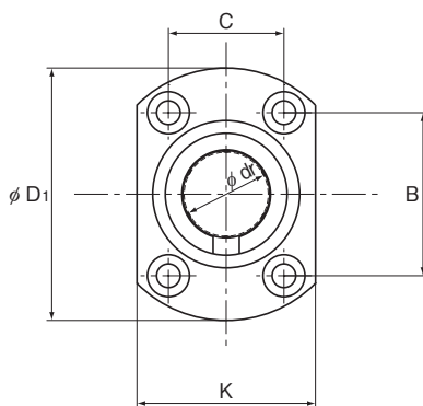
LMIH 16L~25L型
