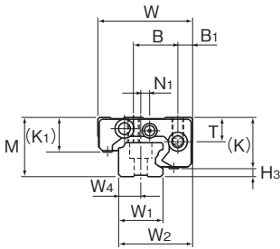
GSR15T/V型
