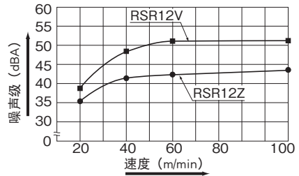
图1 RSR12Z和RSR12V型的噪声级
