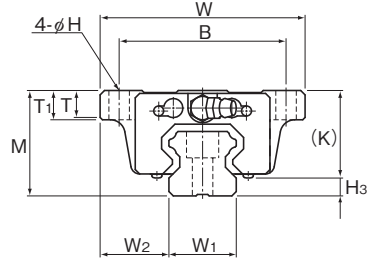
HSR20M1B/M1LB型
