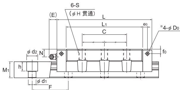
SVS-LC型
