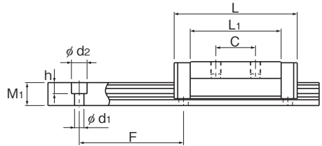
SHW17CRM型、SHW21CRM型
