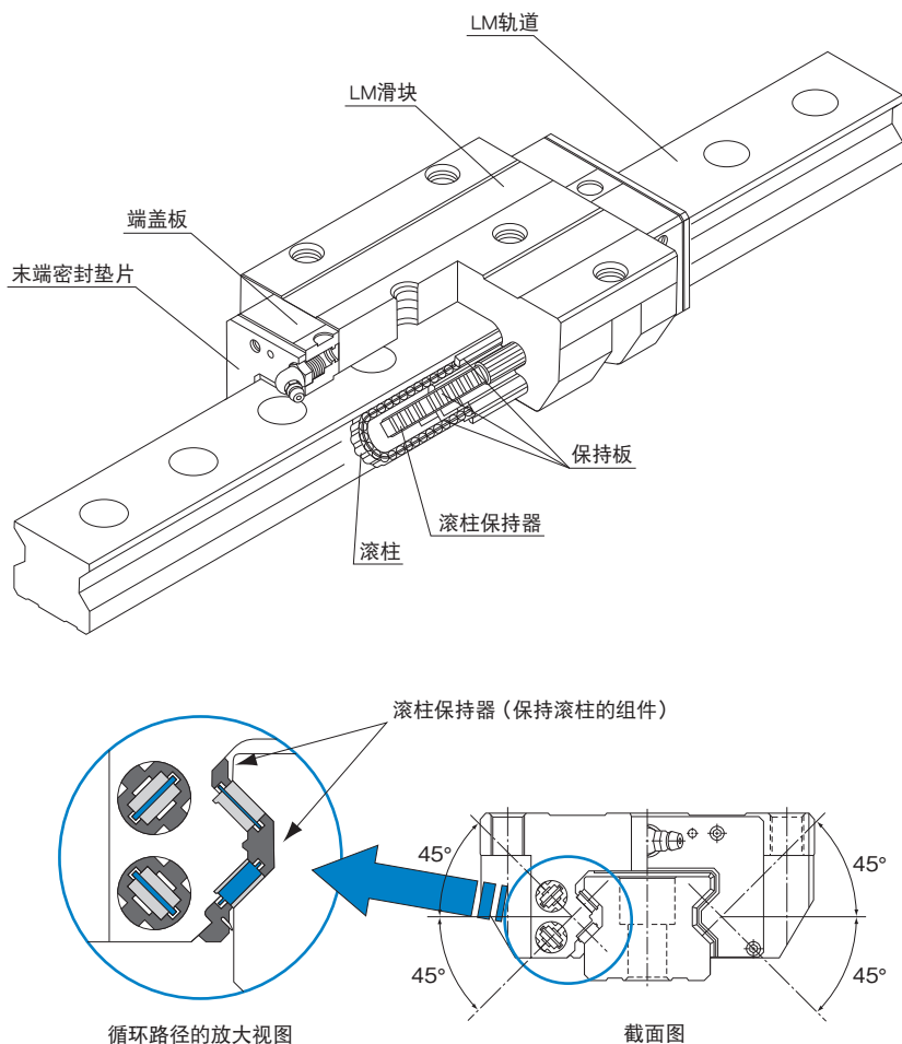
图1 滚柱保持器型LM滚动导轨SRG型的结构图
