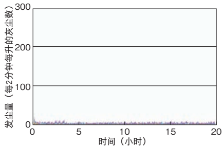
球保持器型LM滚动导轨 SSR20型
