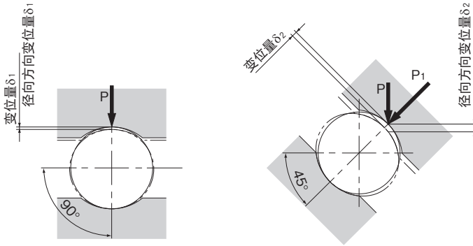
图3 径向载荷下的变位量
