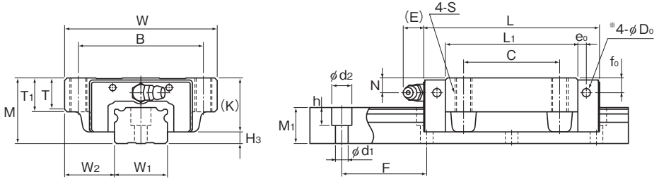
NR-A型
