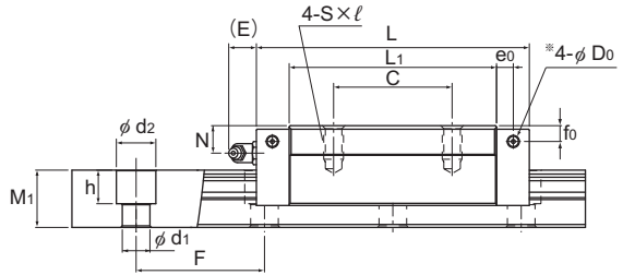
SVS-R型
