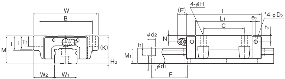
NR-B型
