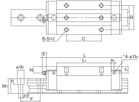
SRG25~65R/LR/LV型
