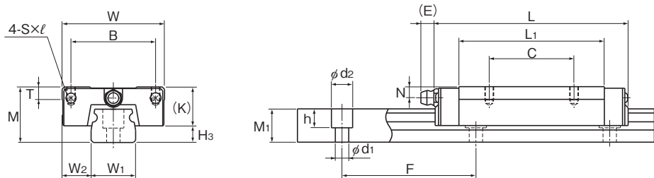
RSR15、20VM/N型
