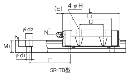
SR-TB型
