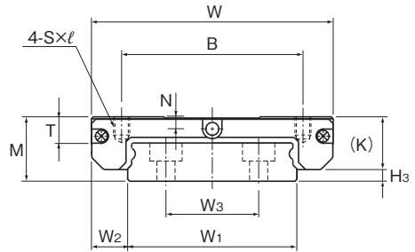
SRS15WM/WN型
