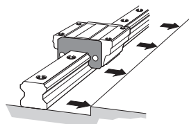
图7 将基准面对上LM轨道
