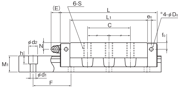
NRS-LA型
