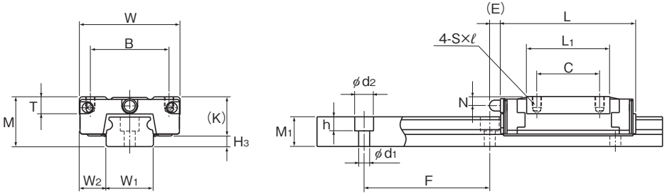
RSR15ZM型
