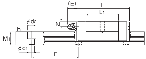
GSR25V-R型
