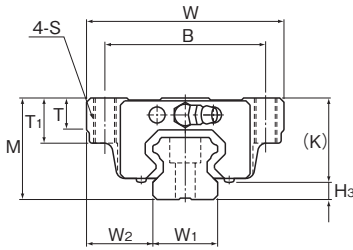
HSR15~35A/LA/AM/LAM型
