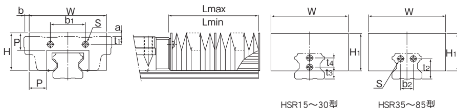
HSR15~30型
