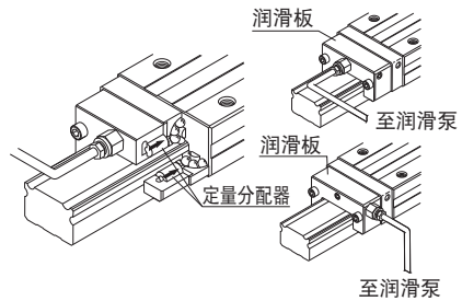
图1 结构图
