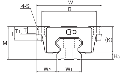
HSR45~85A/LA型
