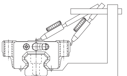
图15 行走平行度
