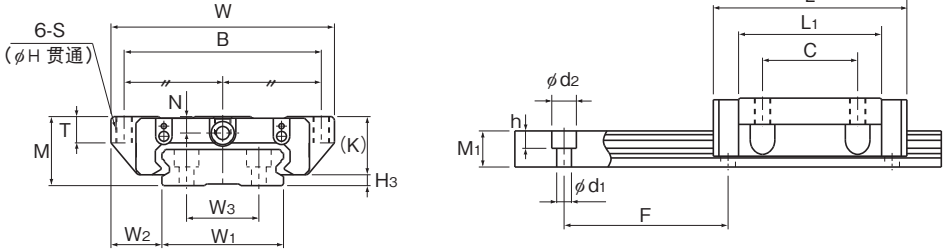
SHW17CAM型、SHW21~50CA型
