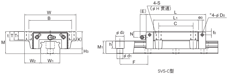
SVS-C型
