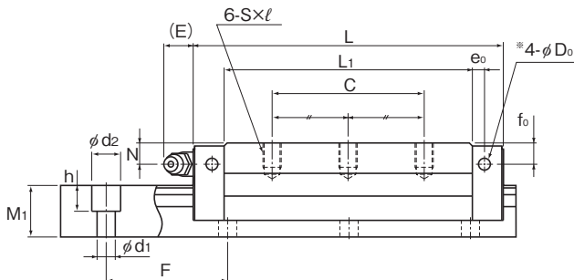
NR-LR型
