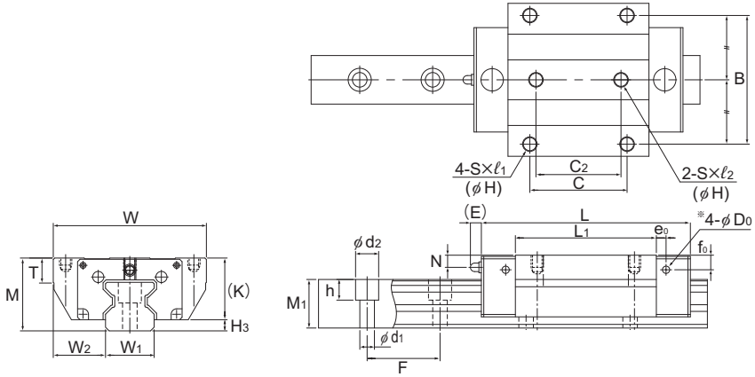
SRG15、20A/LA型
