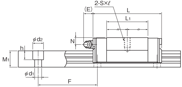
GSR15~25V型
