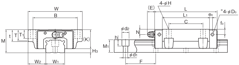
NRS-B型
