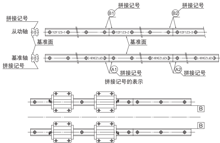
图23 拼接使用
