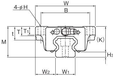
HSR15、25~35M1B/M1LB型
