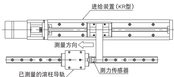
滚动阻力测试装置
