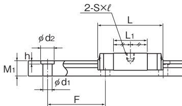
RSR5M/5TN型
