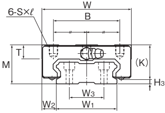
HRW27~50CR/CRM型
