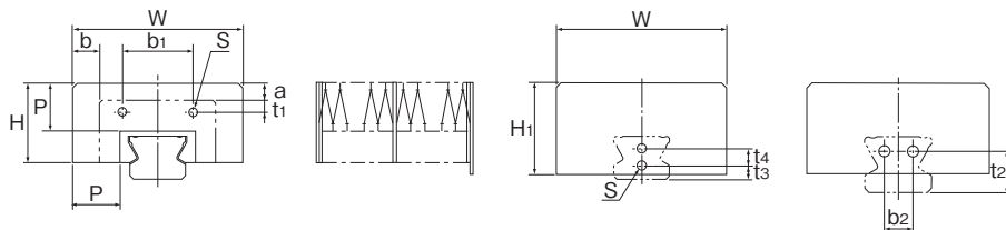
SSR15X~25X型
