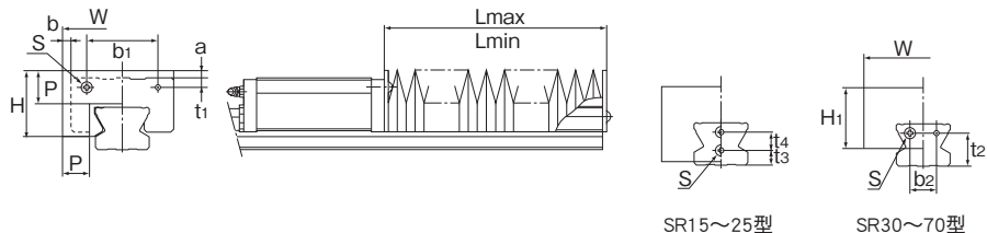
SR15~25型
