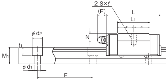
SR-M1V型
