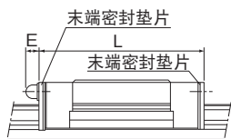
图1 SRS型油嘴的尺寸
