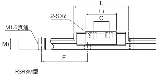
RSR3M型
