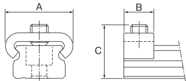
图1 RSR-M1/RSR-M1W型制动器(C型)
