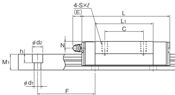
GSR15~35T型
