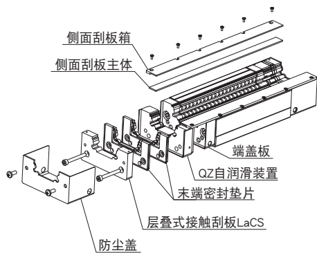
外观图 (例: QZTTHHY型的情况)
