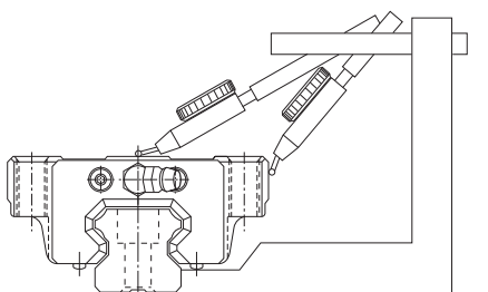
图11 行走平行度
