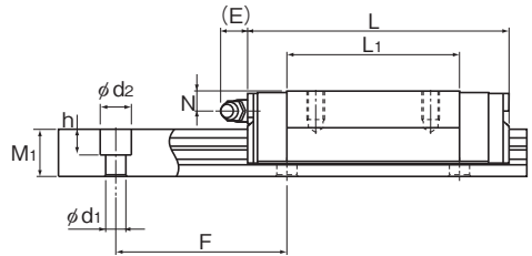
GSR-T-R型
