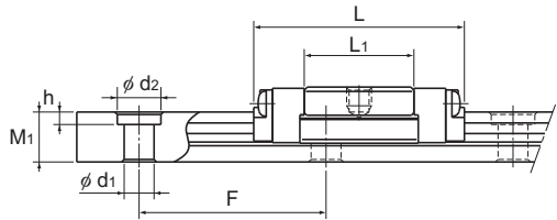
SRS5M型
