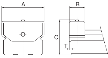
图1 NR/NRS型的末端止动块EP型
