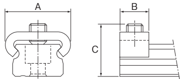
图1 RSR/RSR-W型制动器(C型)
