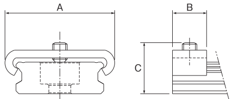
图1 HRW型制动器(C型)
