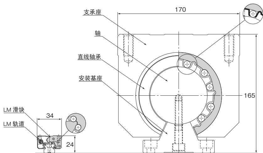
LM 滚动导轨 SSR15XW 型 基本额定载荷：14.7kN
