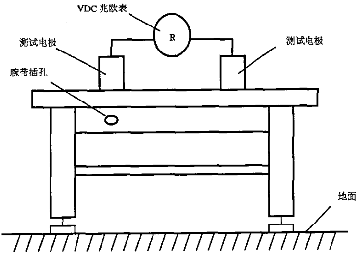
图16 工作台表面点对点电阻测试图
