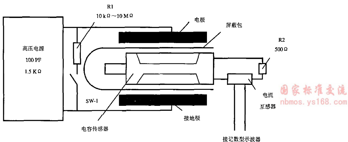
图5 静电屏蔽测试仪原理图
