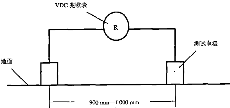
图18 地面点对点电阻测试
