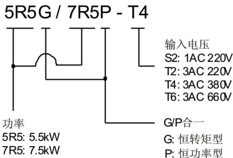
图 2-1 型号说明
