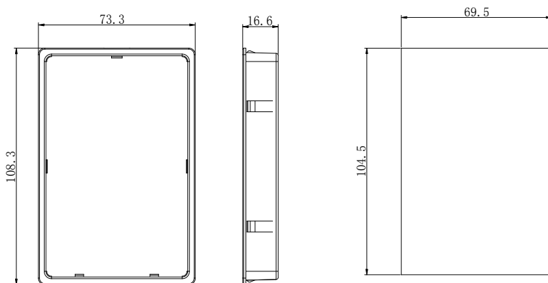
65*100mm 键盘托架尺寸
