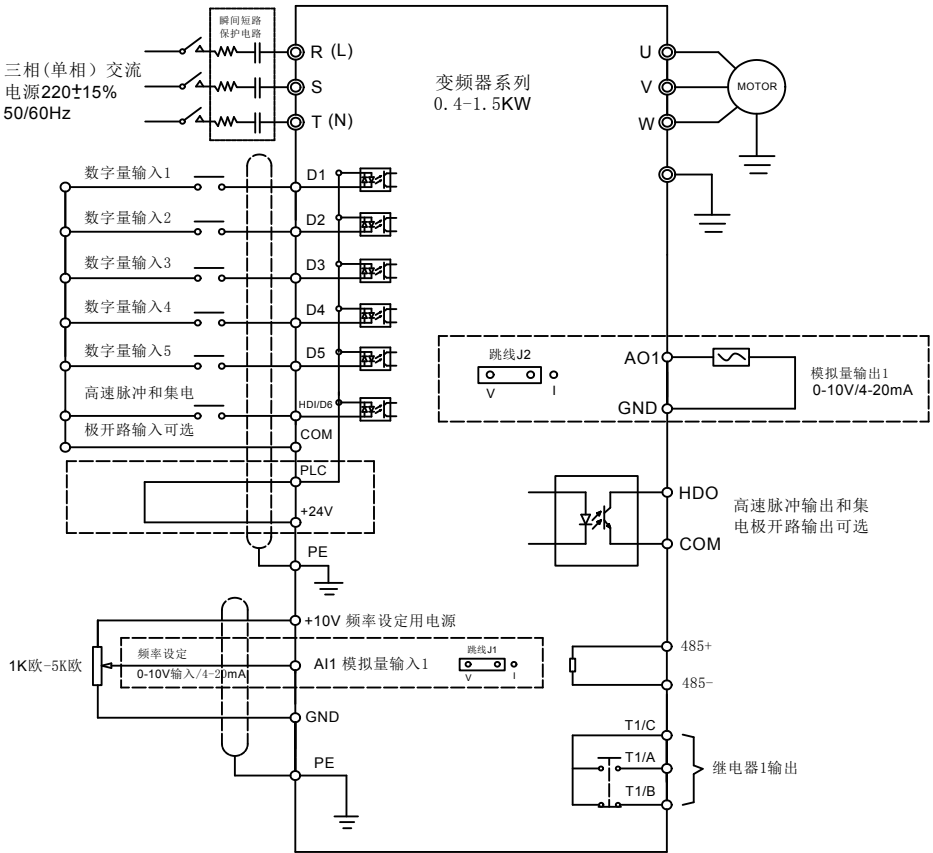
图 3-3 单相/三相 220V 0.4~1.5kW 变频器接线图
