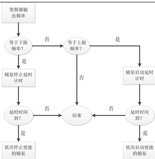
图 6-30 恒压供水逻辑图
