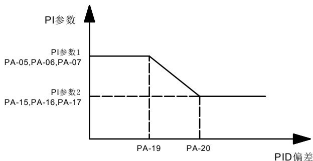
图 6-25 PID 参数切换
