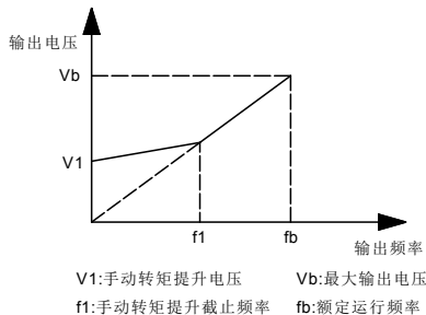
图 6-3 手动转矩提升示意图
