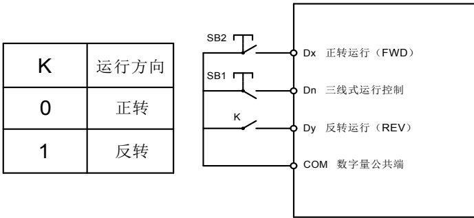
图 6-8 三线式控制模式 2
