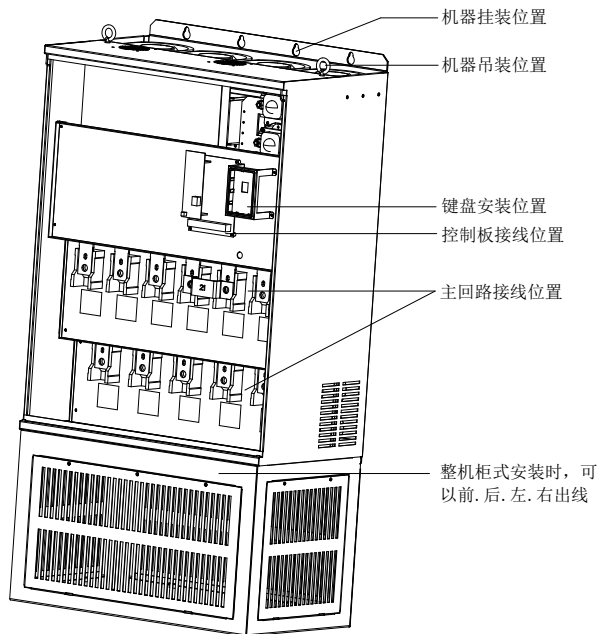
图 2-3 变频器各部件说明
