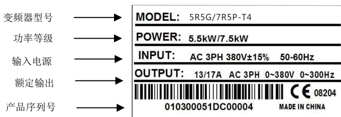
图 2-2 铭牌说明
