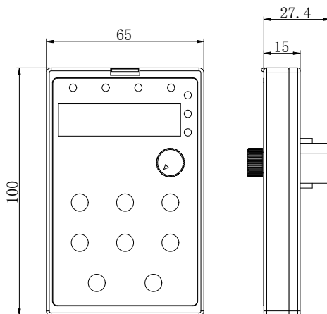
其它功率变频器用 65*100mm 键盘尺寸
