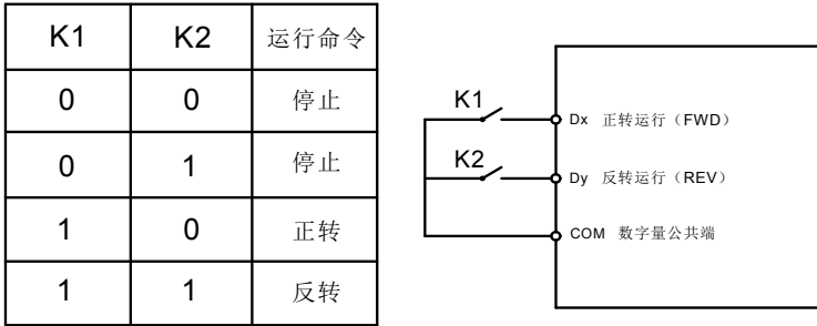
图 6-6 两线式模式 2
