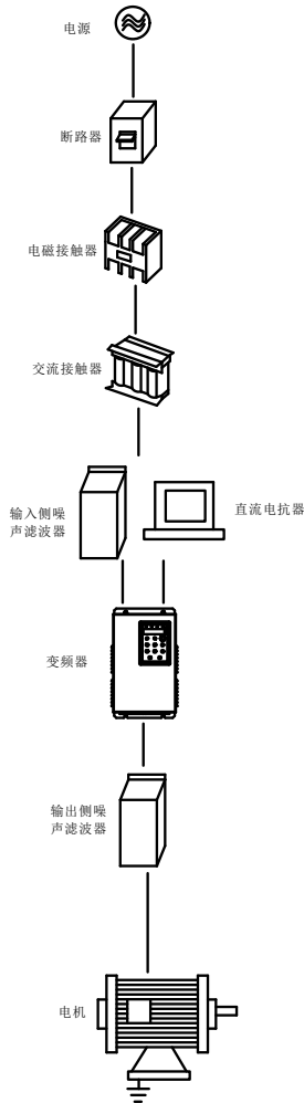
图 3-2 变频器与外围机器的连接示例
