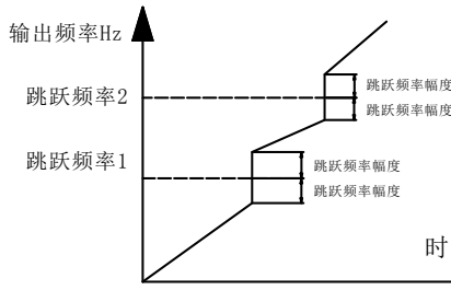
图 6-17 加减速过程中跳跃频率有效示意图
