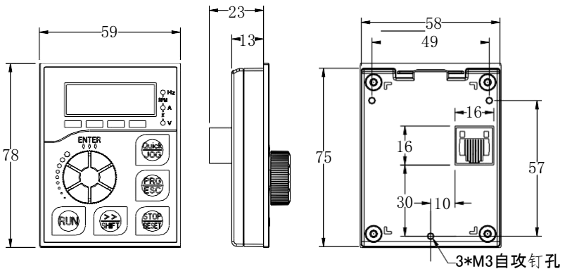
图 2-9.1 小外引键盘不带托盘安装尺寸图
