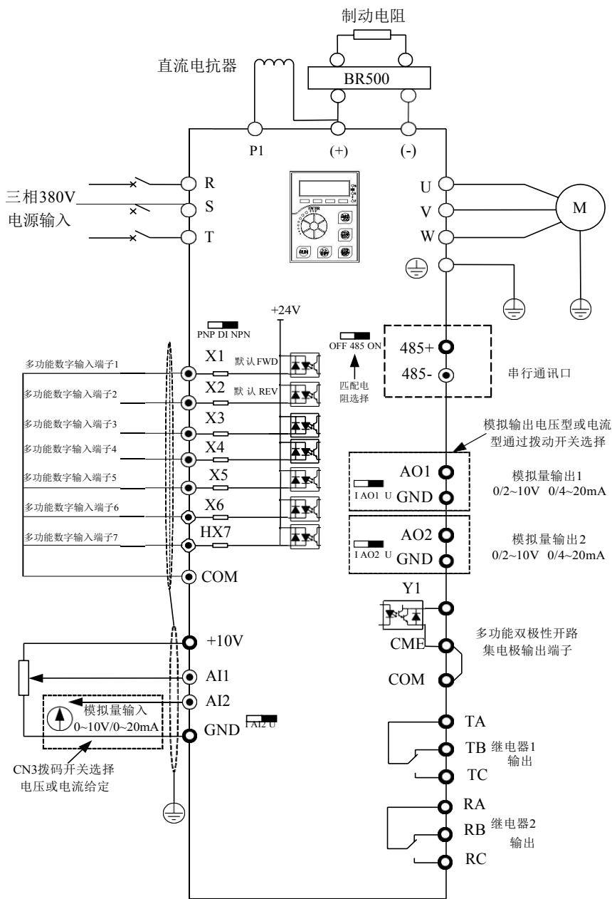
图 3-4. 75Kw (4T:380V 75 Kw) 及以上三相变频器
