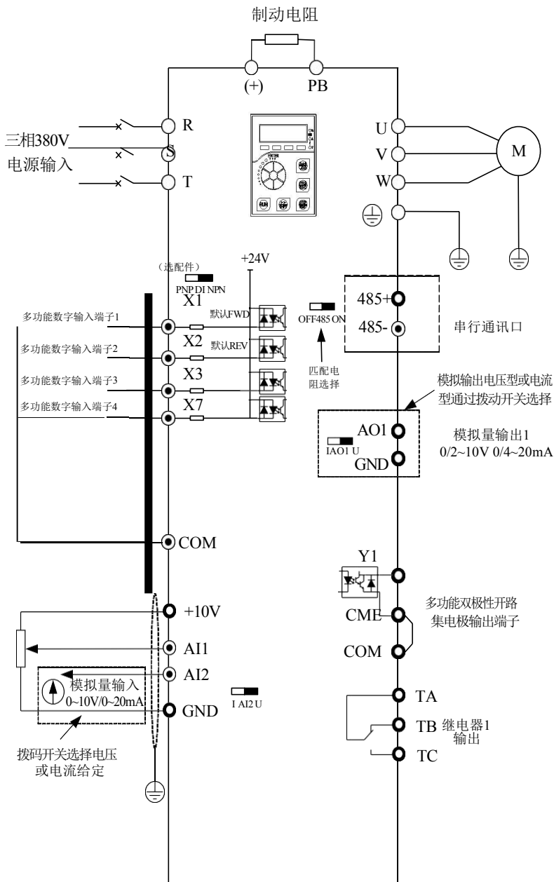
图 3-1. 2.2kW (4T:380V 2.2 kW) 以下三相变频器接线图
