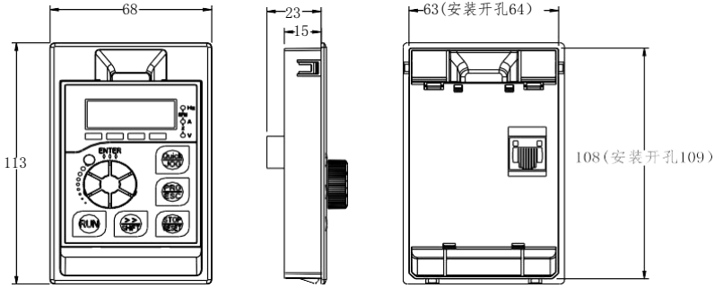
图 2-8.1 小外引键盘带托盘安装尺寸图
