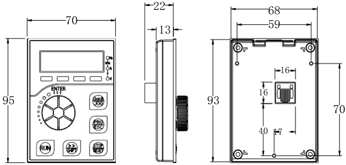
图 2-9.2 大外引键盘不带托盘安装尺寸图
