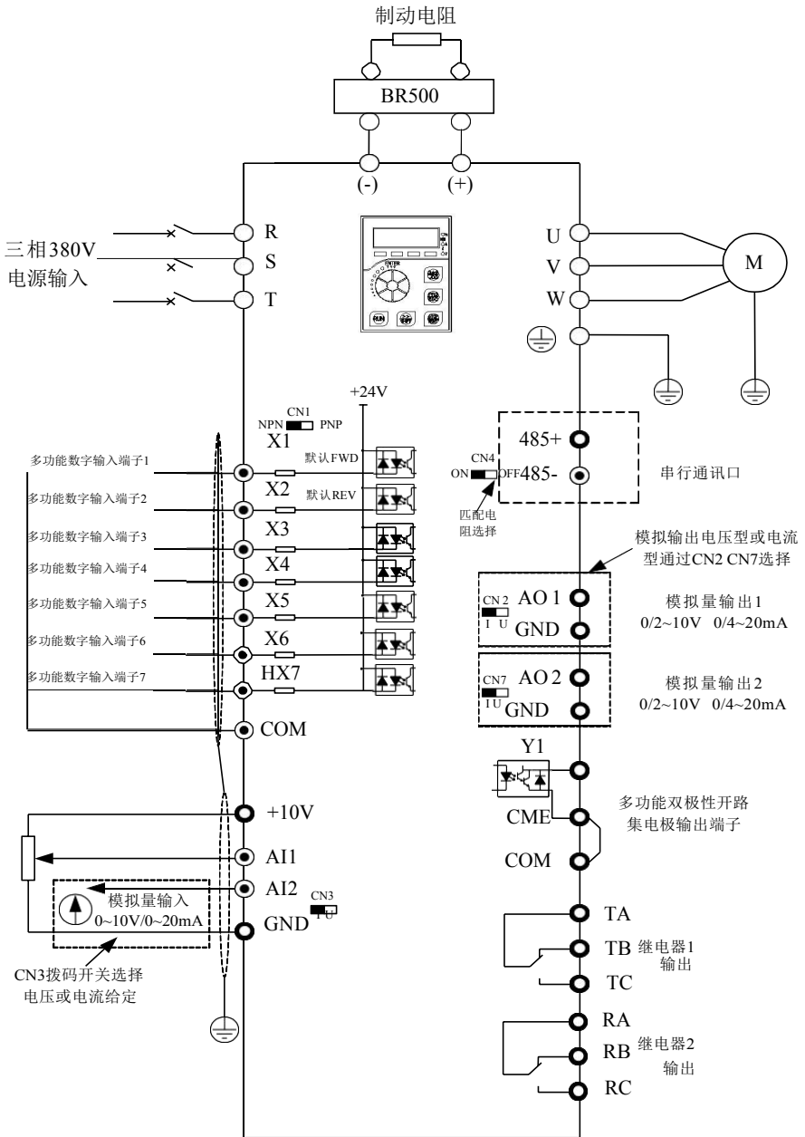
图 3-3.30 ~ 55Kw (4T:380V 30 ~ 55 Kw) 三相变频器不带制动单元功能接线图
