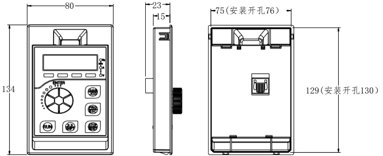
图 2-8.2 大外引键盘带托盘安装尺寸图
